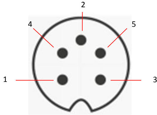
5-pin 240° DIN socket
